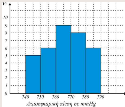
ιστόγραμμα συχνοτήτων
