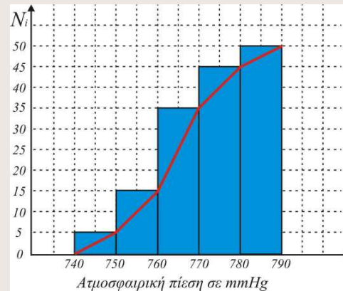
ιστόγραμμα & πολύγωνο αθροιστικών συχνοτήτων
