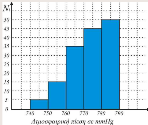
ιστόγραμμα αθροιστικών συχνοτήτων
