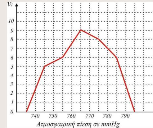
πολύγωνο συχνοτήτων
