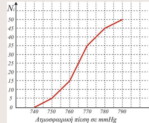
πολύγωνο αθροιστικών συχνοτήτων
